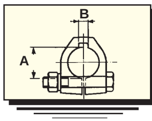
MACHOIRES ALESEES AVEC RAINURE DE CLAVETTE ET BOULON SECANT PLAIN BORE YOKES WITH KEYWAY AND INTERFERING BOLT
