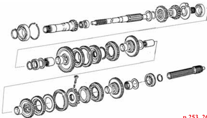
p 253, 267 Arbre primaire / Mainshaft
