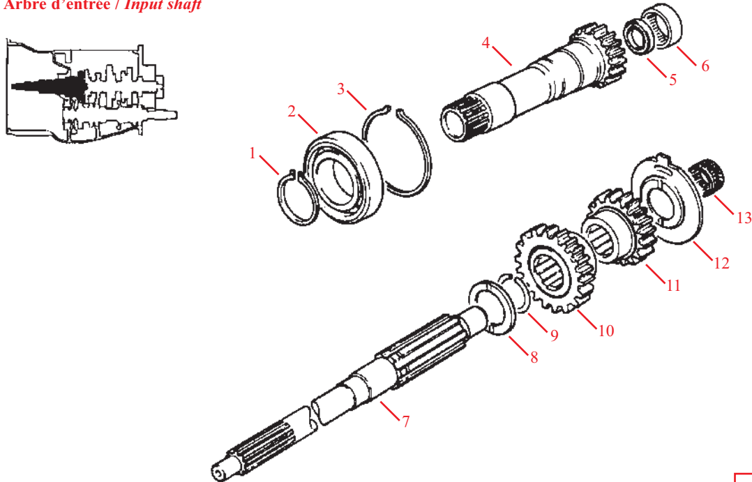
Arbre d'entrée / Input shaft
