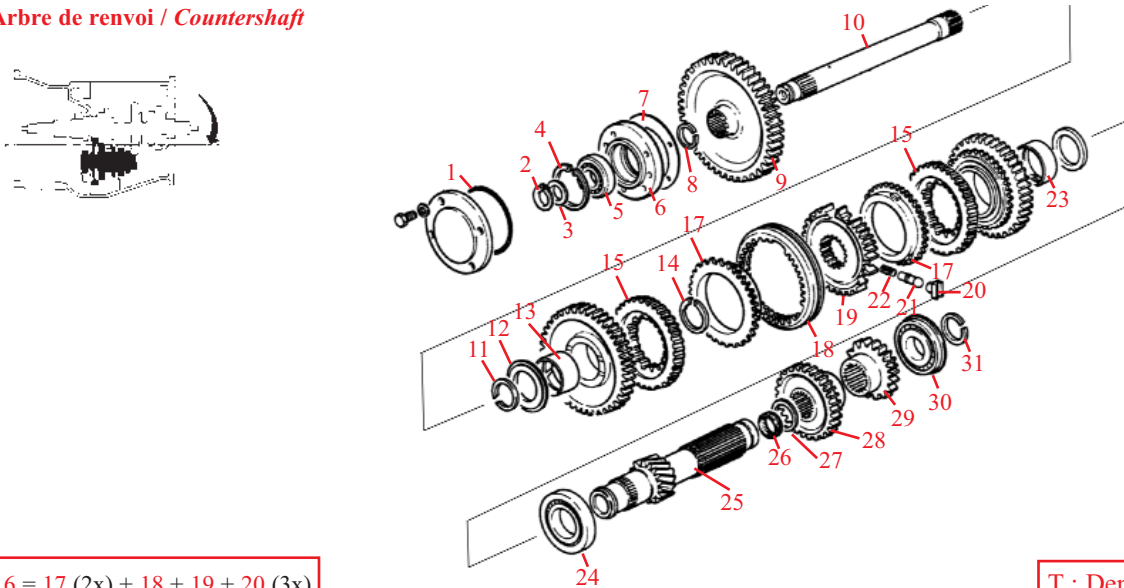
Arbre de renvoi / Countershaft
